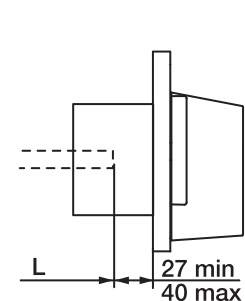
Door clutch ONZ45P
