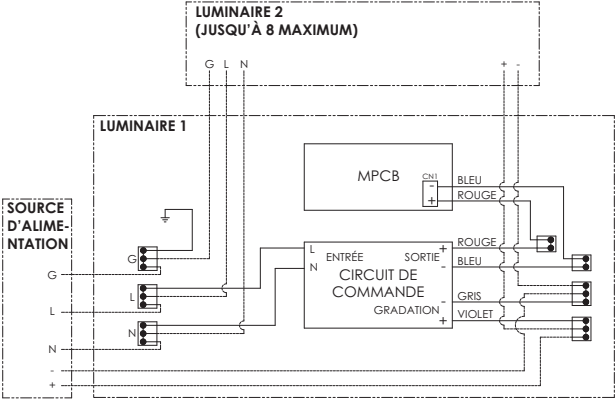
PASSAGE DE CÂBLAGE D'ALIMENTATION
