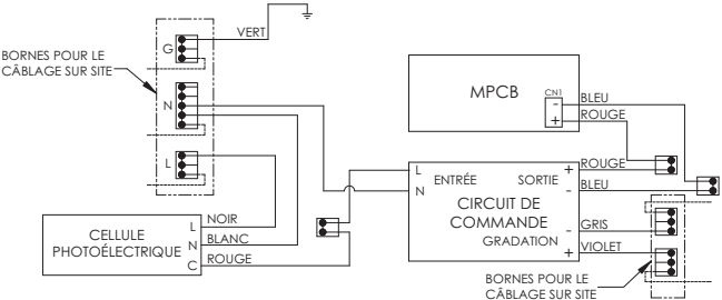
CÂBLAGE DE LA CELLULE PHOTOÉLECTRIQUE
