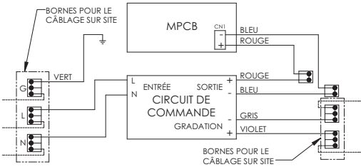
CÂBLAGE STANDARD
