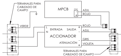
CABLEADO ESTÁNDAR
