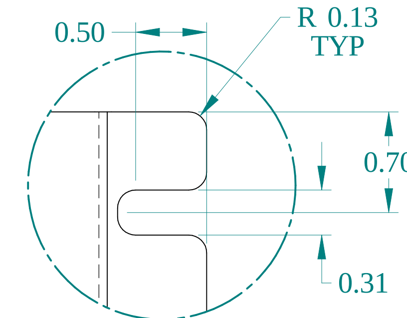
DETAIL Z TYP (4)
