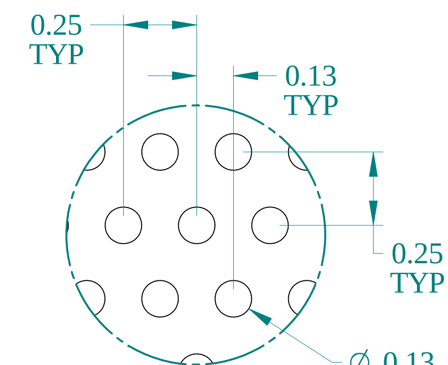
DETAIL Y
