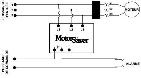
(B) Pour déclencher une alarme : Brancher le contact normalement fermé en série avec l'alarme, tel qu'illustré.
