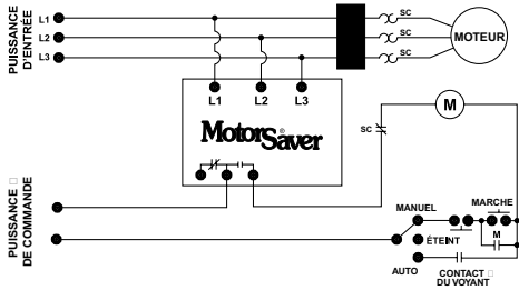
(A) Pour commander un moteur : Brancher le contact normalement ouvert en série avec la bobine magnétique du démarreur de moteur, tel qu'illustré.
