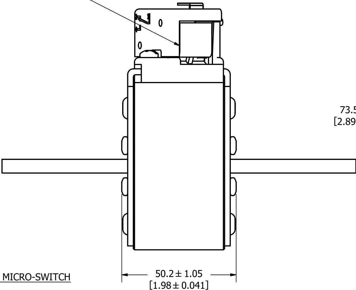
VISUAL INDICATOR
