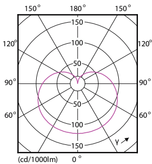
Light Distribution Diagram - 14A19/COR/927/FR/P/E26/DIM/T20 6/1CT
