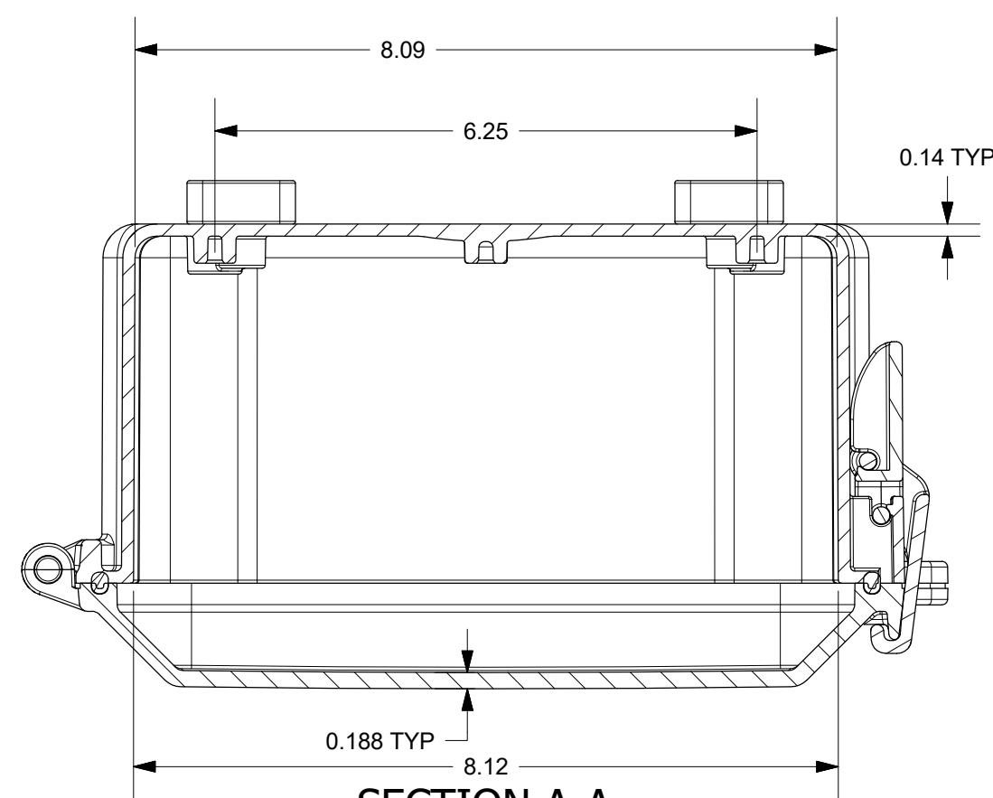
SECTION A-A
