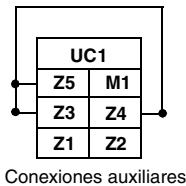
Figura 33 – Terminales en puente
