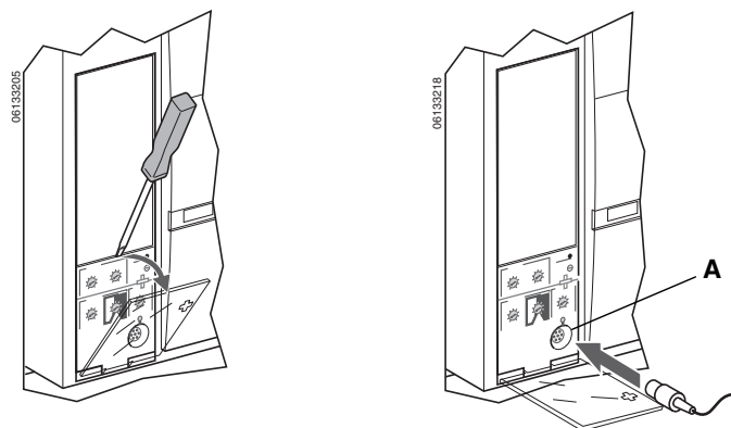
Figure 37 – Vérification du fonctionnement du déclencheur
