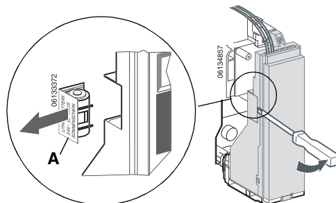
Figure 51 – Enlever le couvercle de la pile
