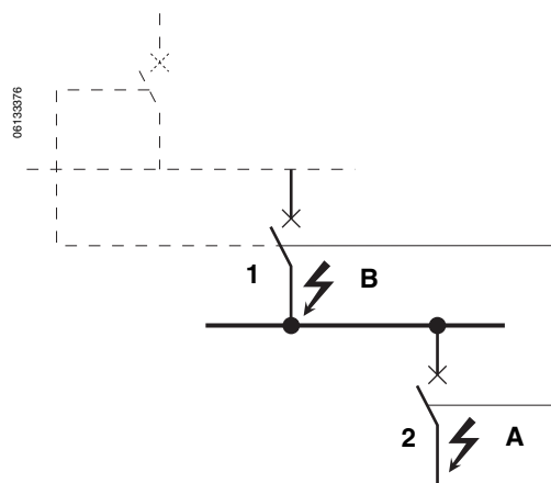
Figure 6 – Interlocking sélectif de zone
