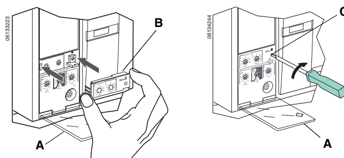
Figure 48: Instalación del calibrador ajustable
