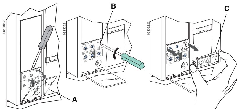
Figure 41 – Retrait de la fiche de valeur nominale réglable
