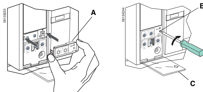
Figure 49 – Installer la nouvelle fiche de valeur nominale réglable
