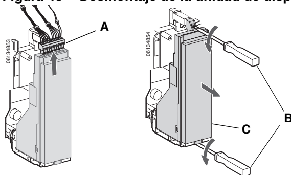
Figura 43 – Desmontaje de la unidad de disparo existente
