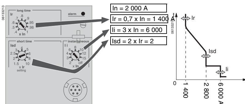
Figure 29 – Régler les niveaux d'enclenchement
