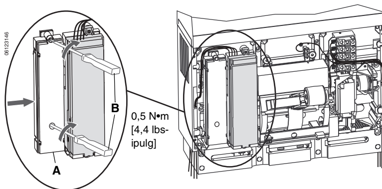
Figura 54 – Colocación del módulo de aguate
