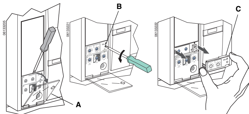
Figura 49 – Extracción del calibrador ajustable
