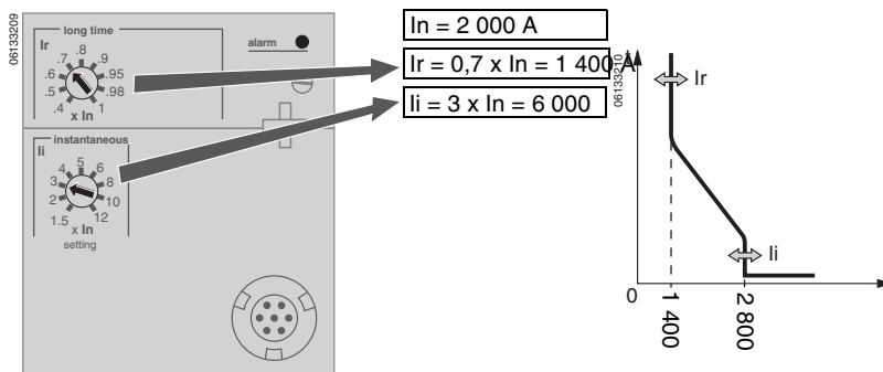
Figura 27 – Ajuste de los niveles de activación
