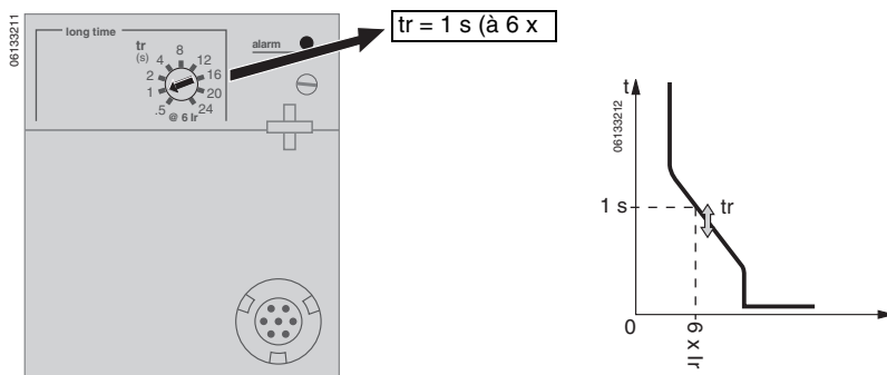
Figure 28 – Régler la temporisation
