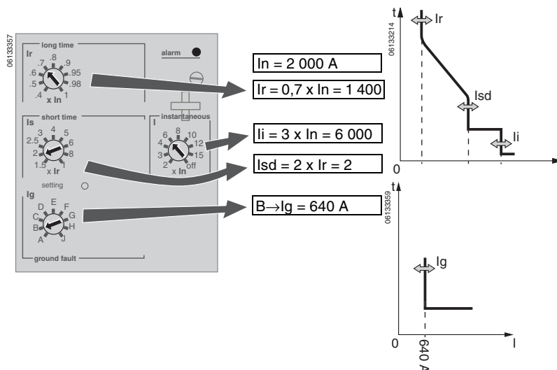
Figure 31 – Régler les niveaux d'enclenchement
