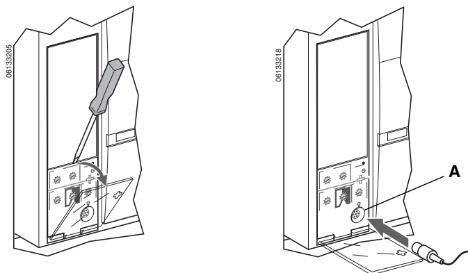
Figura 38 – Verificación del funcionamiento de la unidad de disparo
