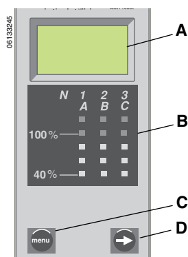
Figure 14 – Ampèremètre
