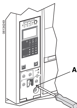
Figure 38 – Vérification des fonctions de déclenchement d'appareil sur défaut à la terre
