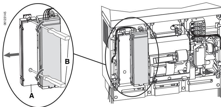
Figura 51 – Desplazamiento del módulo de aguate
