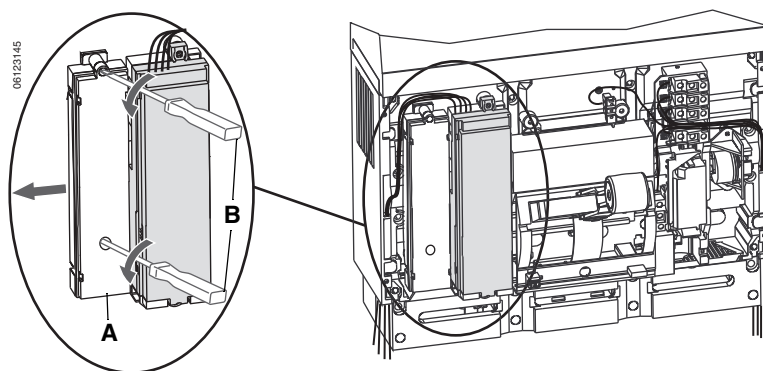
Figure 50 – Déplacer le module de tenue
