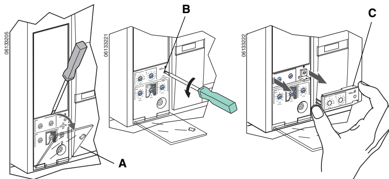
Figura 42 – Desmontaje del calibrador ajustable
