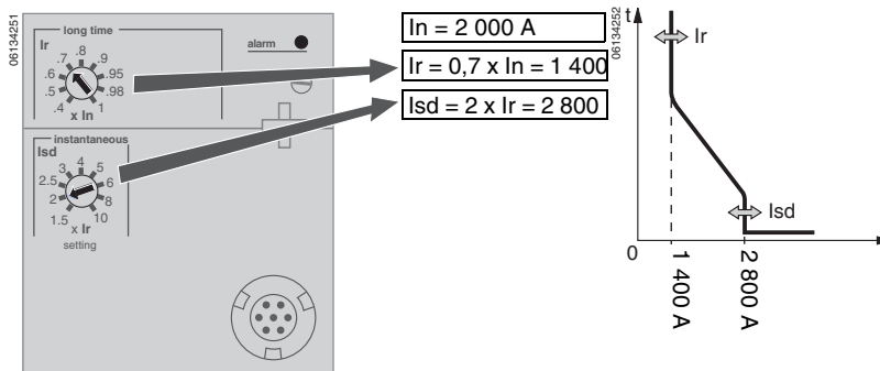
Figura 25 – Ajuste de los niveles de activación
