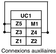
Figure 33 – Bornes reliées par cavalier
