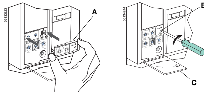
Figura 50 – Instalación del nuevo calibrador ajustable
