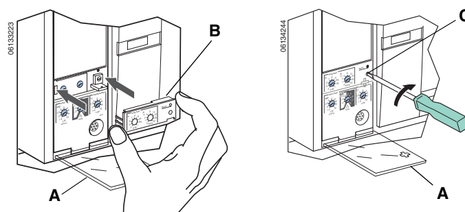
Figure 47: Installation de la fiche de valeur nominale réglable
