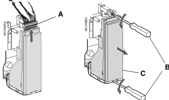
Figure 42 – Retrait du déclencheur existant
