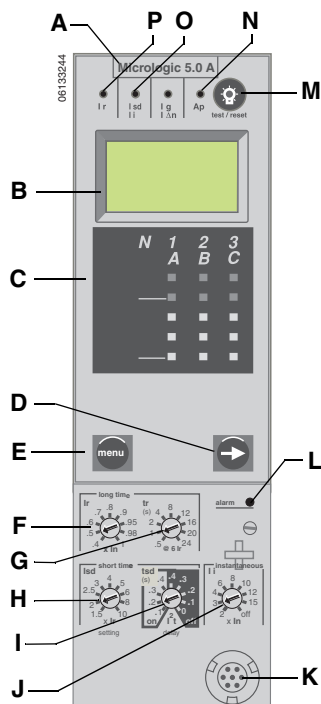
Figura 4 – Unidad de disparo 5.0A
