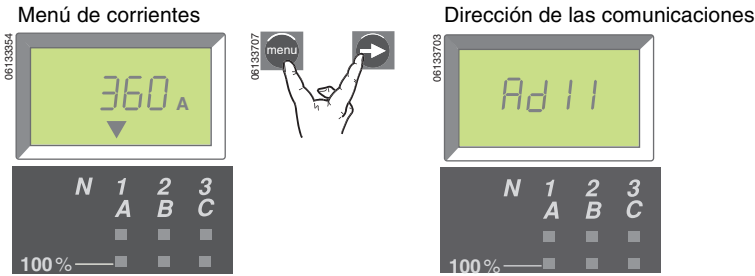
Figura 35 – Acceso al menú del módulo de comunicación
