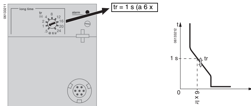
Figura 28 – Ajuste del retardo de tiempo
