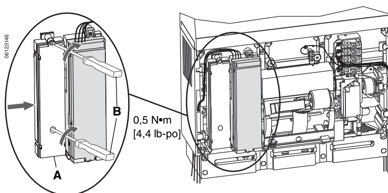
Figure 53 – Replacer le module de tenue
