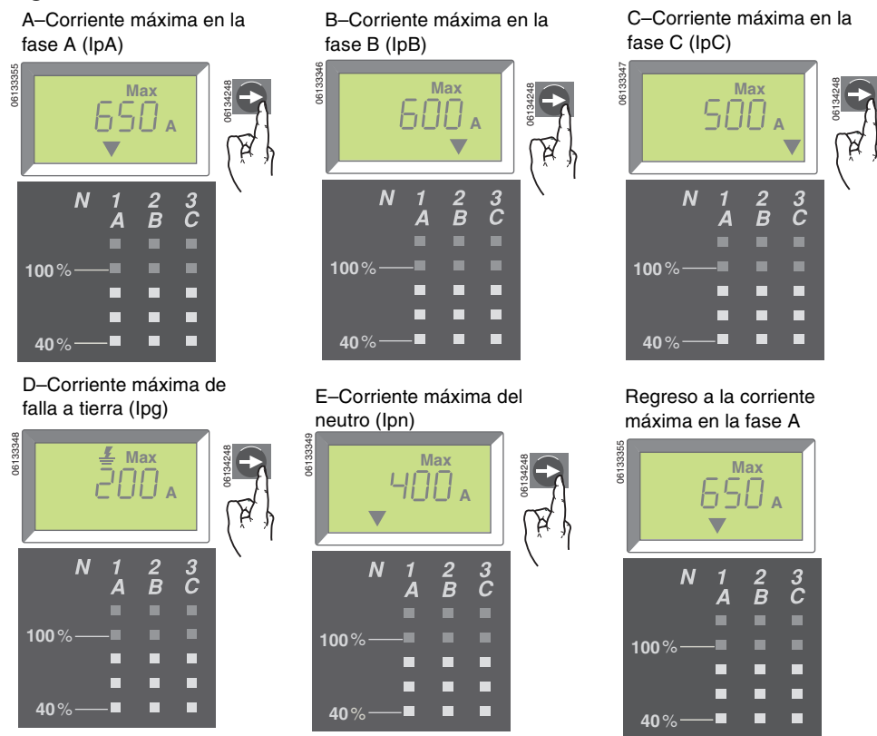
Figura 19 – Corrientes máximas
