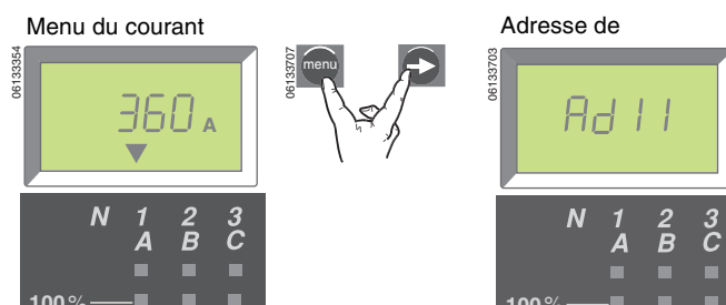
Figure 35 – Accès au menu du module de communication
