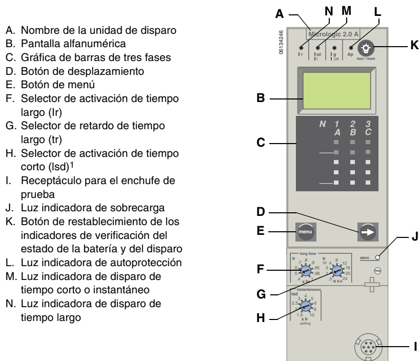
Figura 2 – Unidad de disparo 2.0A
