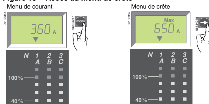
Figure 18 – Accès au menu de crête
