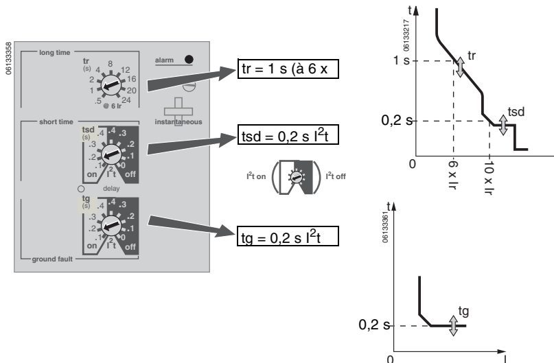
Figure 32 – Régler les temporisations
