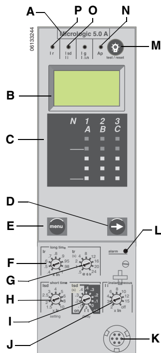
Figure 4 – Déclencheur 5.0A
