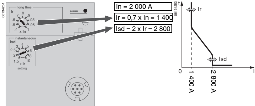
Figure 25 – Régler les niveaux d'enclenchement
