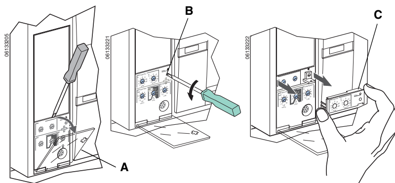
Figure 48 – Enlever la fiche de valeur nominale réglable
