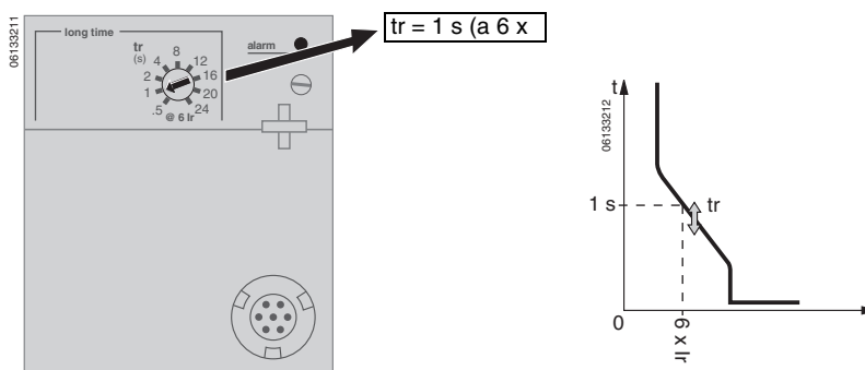
Figura 26 – Ajuste del retardo de tiempo
