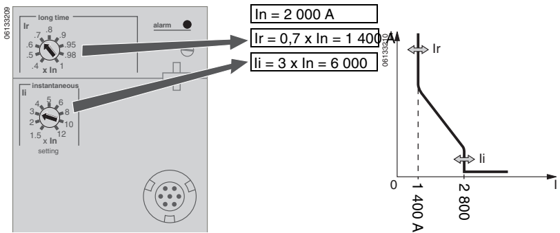
Figure 27 – Régler les niveaux d'enclenchement
