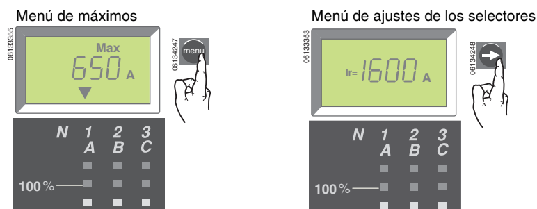
Figura 20 – Acceso a los ajustes de los selectores
