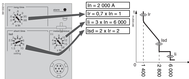
Figura 29 – Ajuste de los niveles de activación
