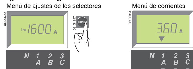
Figura 22 – Regreso al menú de corrientes
