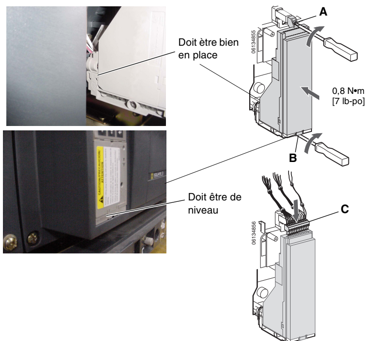
Figure 46 – Installation du déclencheur
