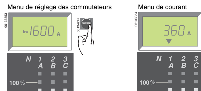
Figure 22 – Revenir au menu de courant
