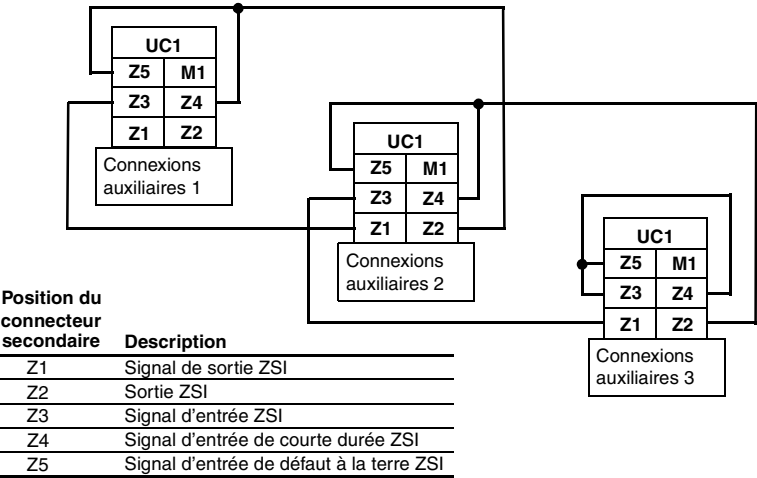
Figure 34 – Exemple de câblage ZSI
