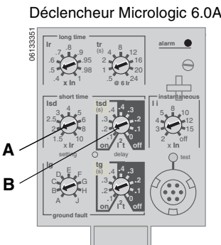
Figure 10 – Commutateurs de protection contre les défauts à la terre
