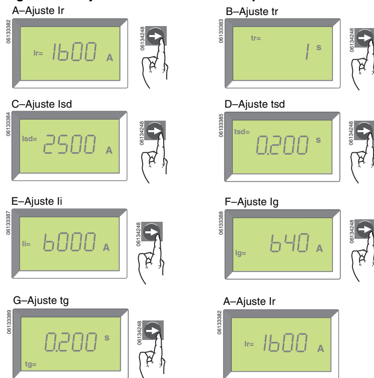
Figura 21 – Ajustes de la unidad de disparo
