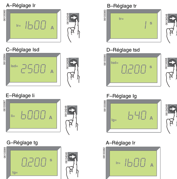
Figure 21 – Réglages du déclencheur
