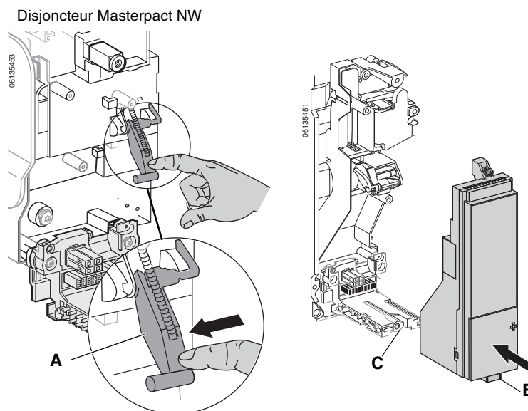
Figure 45 – Installation du déclencheur
