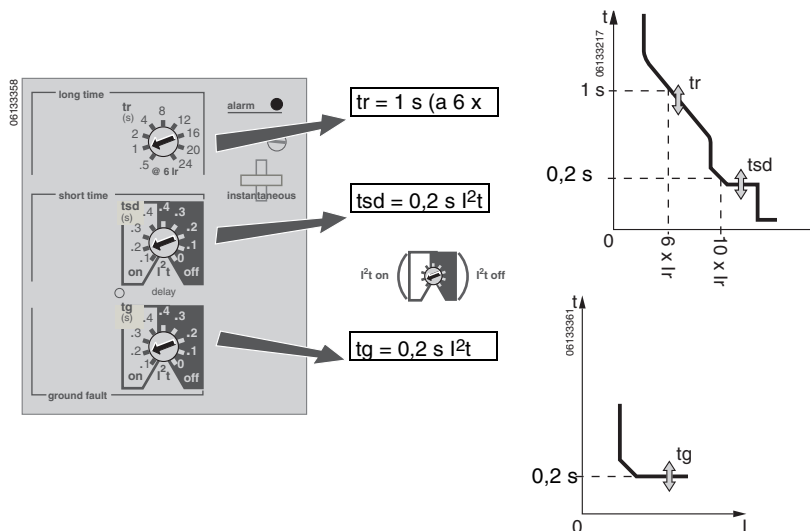
Figura 32 – Ajuste del retardo de tiempo
