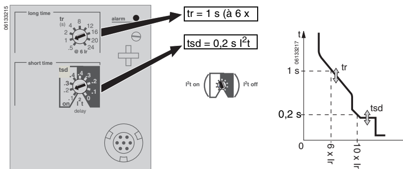
Figure 30 – Régler les temporisations
