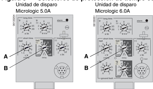
Figura 8 – Selectores de protección de tiempo corto
