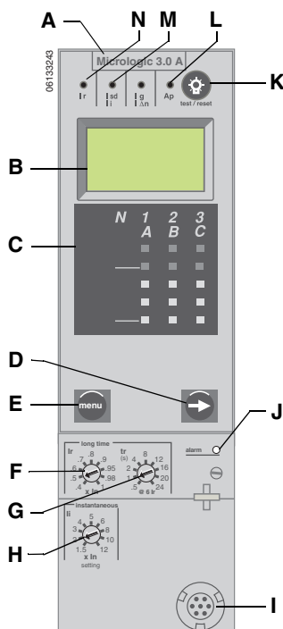
Figure 3 – Déclencheur 3.0A
