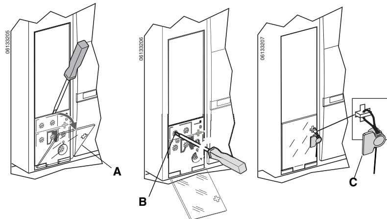
Figure 23 – Réglage des commutateurs
