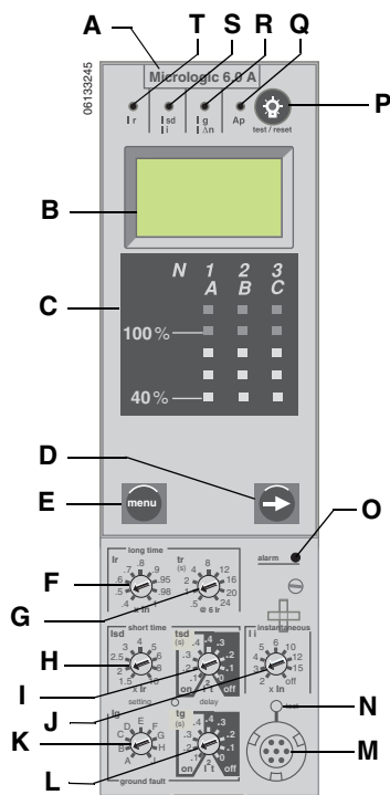
Figure 5 – Déclencheur 6.0A
