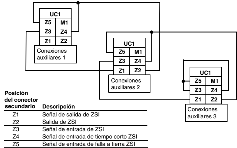
Figura 34 – Ejemplo de cableado de ZSI
