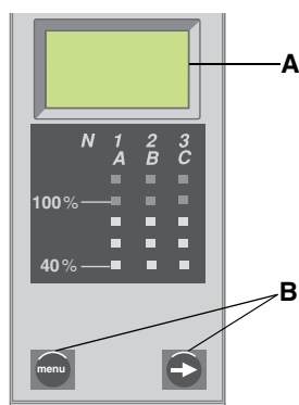
Figura 13 – Ampérmetro
