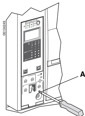
Figura 39 – Prueba de las funciones de disparo por falla a tierra del equipo
