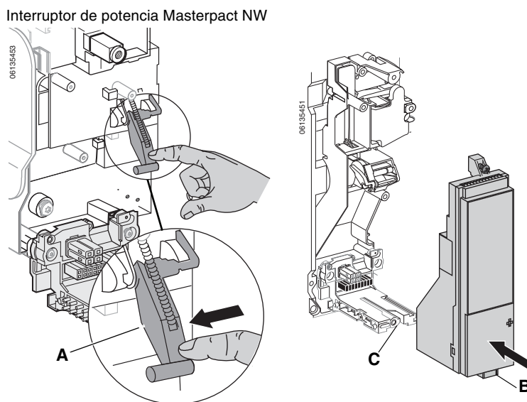
Figura 46 – Instalación de la unidad de disparo
