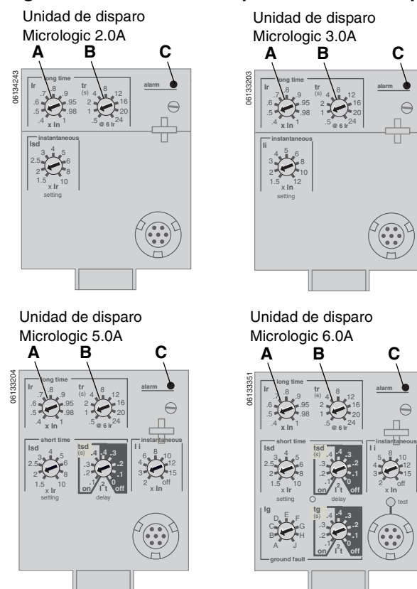
Figura 7 – Selectores de protección de tiempo largo
