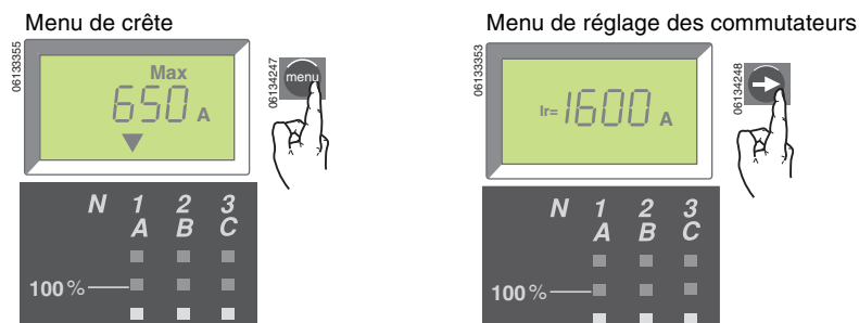
Figure 20 – Accès au menu de réglage des commutateurs
