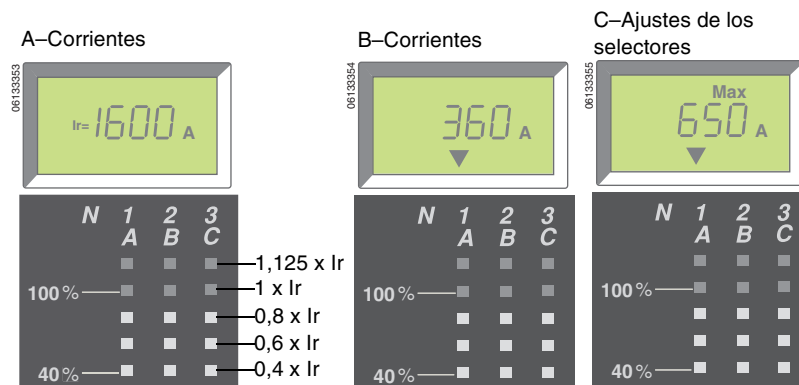
Figura 15 – Menús
