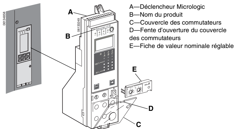
Figure 1 – Déclencheur Micrologic
