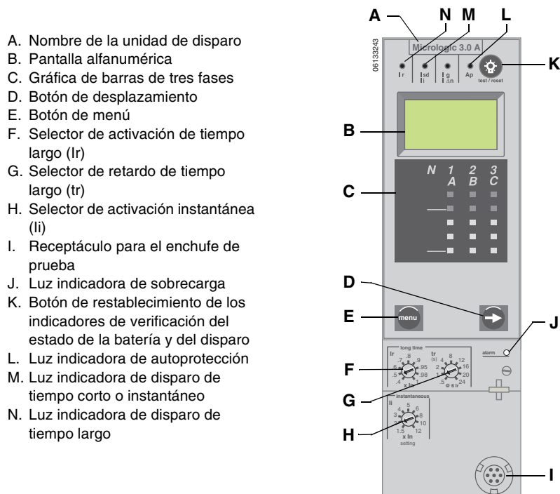
Figura 3 – Unidad de disparo 3.0A
