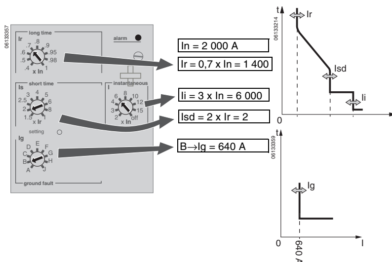
Figura 31 – Ajuste de los niveles de activación
