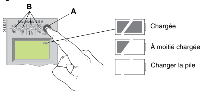
Figure 40 – Vérification de l'état du déclencheur
