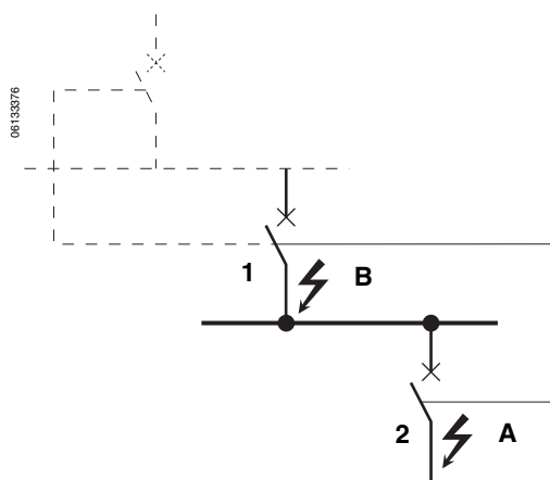
Figura 6 – Enclavamiento selectivo de zona
