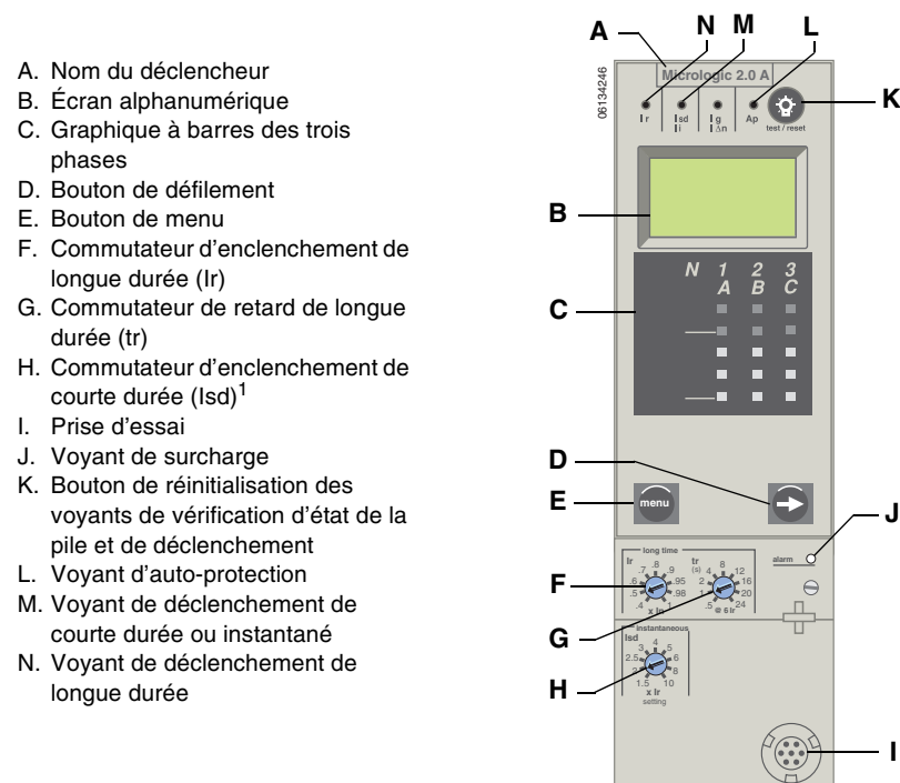
Figure 2 – Déclencheur 2.0A
