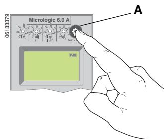
Figure 39 – Réarmement du déclencheur
