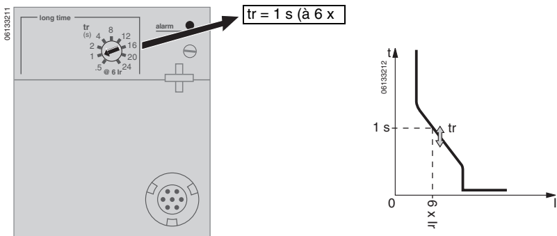
Figure 26 – Régler la temporisation
