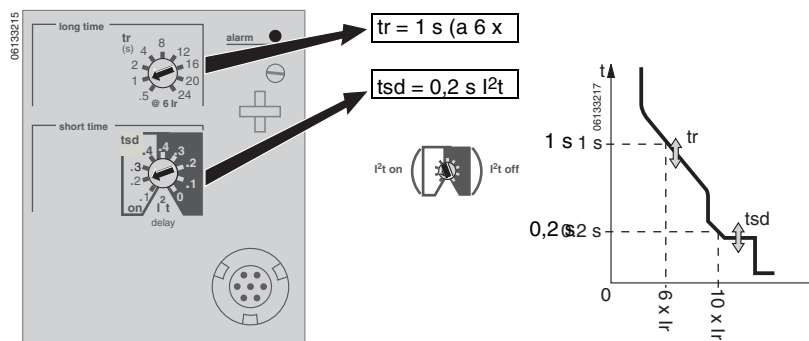
Figura 30 – Ajuste del retardo de tiempo
