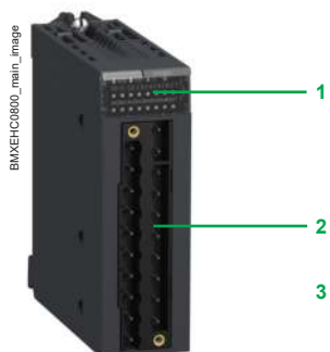
BMXEHC0800
