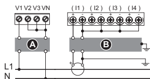
1PH2W LN
