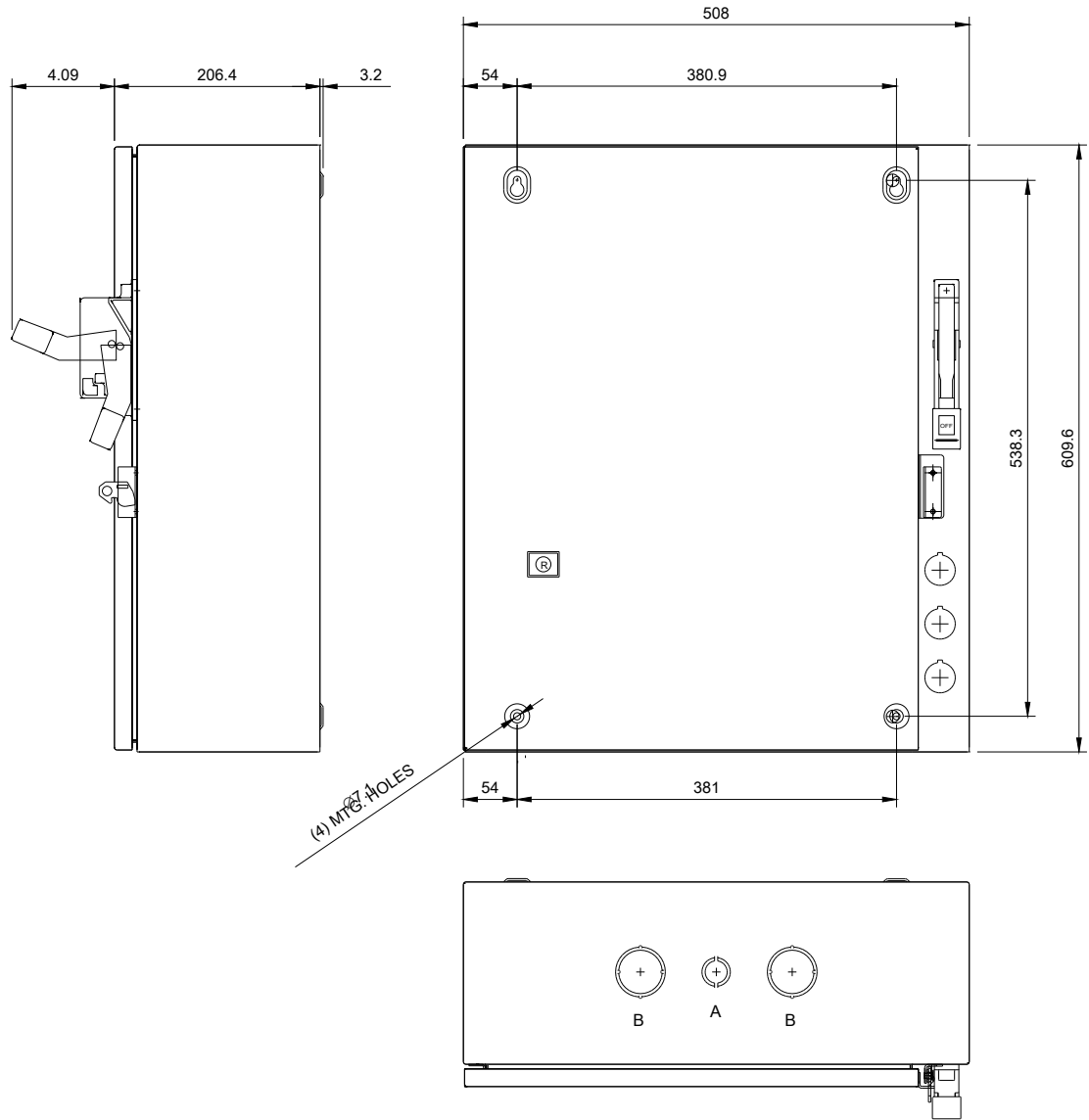
1\CONDUITS TYP. TOP & BOTTOM
