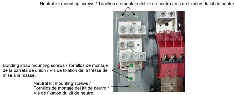
Figure / Figura / Figure 1 : 400 A and 600 A Neutral / Neutro de 400 A y 600 A / Neutre à 400 A et 600 A
