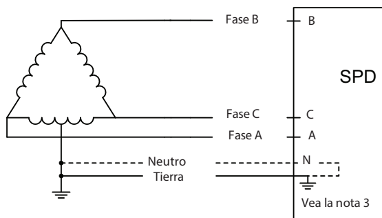
Figura 7: Instalación en delta de tres fases, tres hilos + tierra
