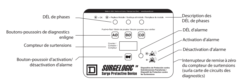
Figure 10 : Panneau de surveillance des diagnostics triphasé avec compteur de surtensions
