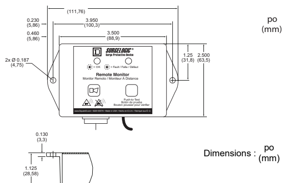
Figure 12 : Option de moniteur à distance (TVS12RMU)
