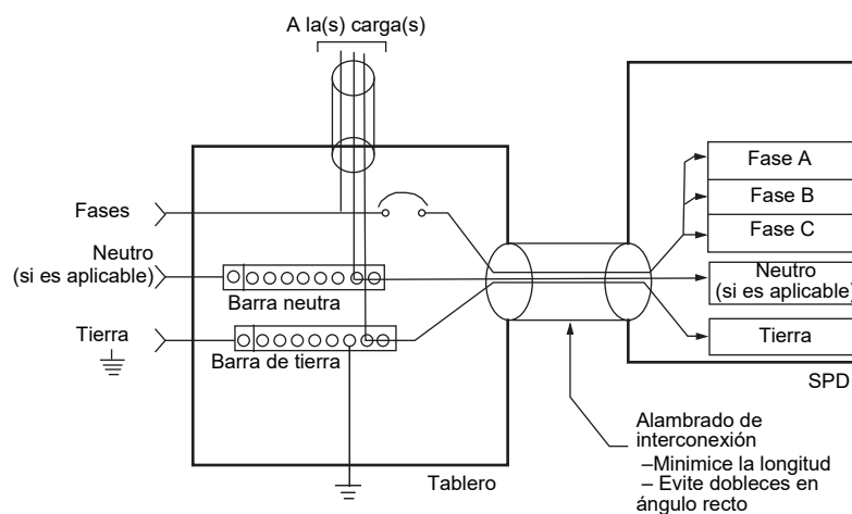
Figura 2 – Prácticas de alambrado del dispositivo de protección contra sobretensiones transitorias
