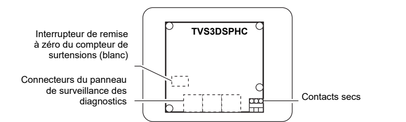
Figure 11 : Arrière de la carte de circuits des diagnostics
