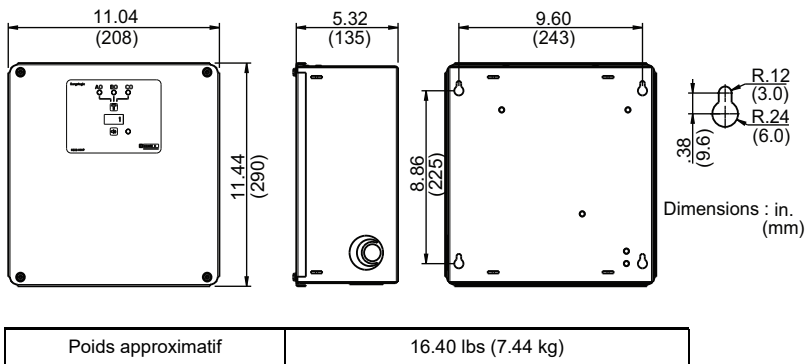
Figure 3 : Coffrets NEMA 1 de 11 x 12 po
