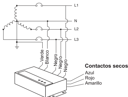
Figura 7 – Instalación en delta con extremo alto de tres fases, 3 ó 4 hilos
