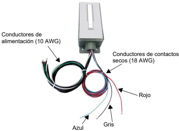
Figura 13: Conductores
