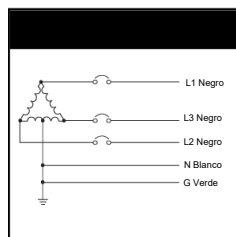
Figura 9: Instalación en delta con extremo alto trifásica, 3 ó 4 hilos 2
