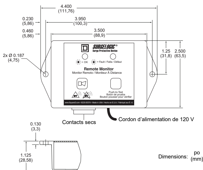
Figure 14 : Option de moniteur à distance (TVS12RMU)
