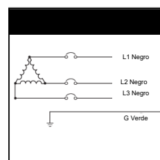
Figura 10: Instalación en delta trifásica, 3 hilos
