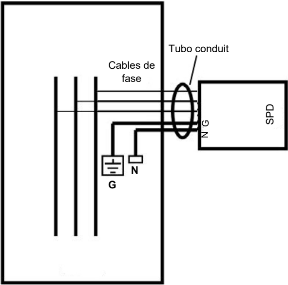
Figure 5: Diagrama de cableado paralelo
