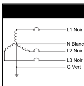
Figure 9 : Installation en sommet de triangle triphasée, à 3 ou 4 fils 2
