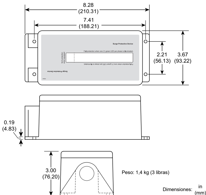
Figura 11: Dimensiones generales
