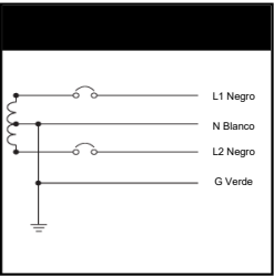
Figura 6: Instalación con conexión a tierra monofásica, tres hilos
