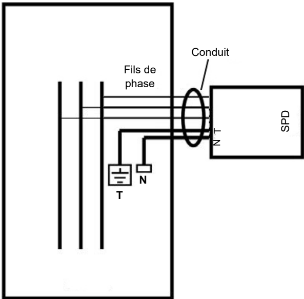
Figure 5: Schéma de câblage en parallèle
