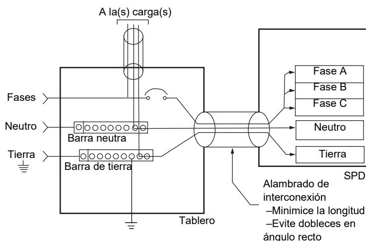
Figura 2: Alambrado del SPD para las configuraciones en delta con extremo alto y en estrella
