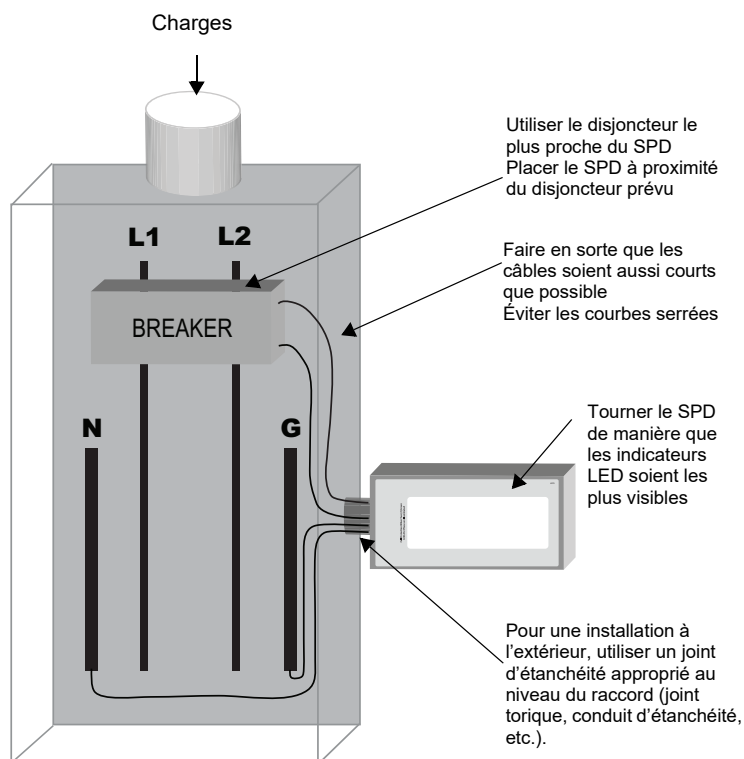
Figure 4 : Installation typique du panneau
