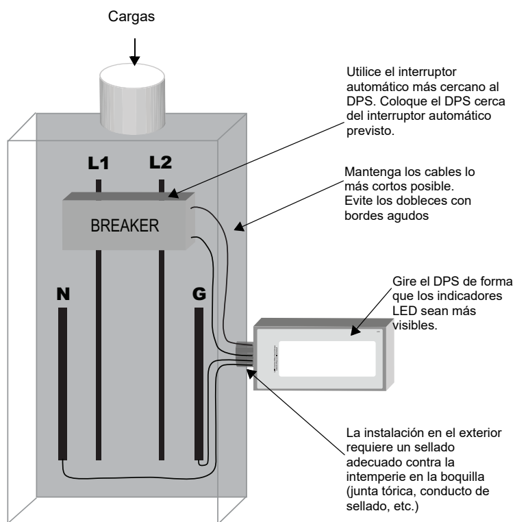
Figura 4: Instalación típica del tablero
