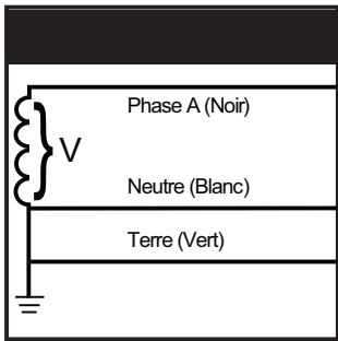
Figure 7 : Monophasé, deux fils, mise à la terre
