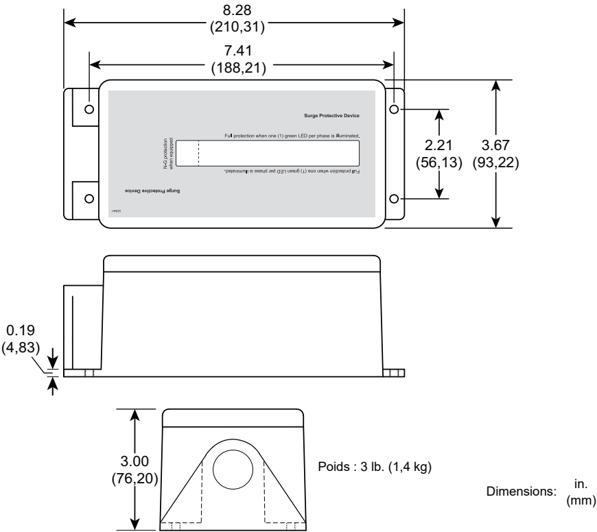
Figure 11 : Dimensions générales
