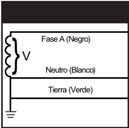
Figura 7: Monofásica, dos hilos, tierra
