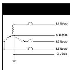
Figura 8: Instalación en estrella con conexión a tierra trifásica, 3 o 4 hilos 1
