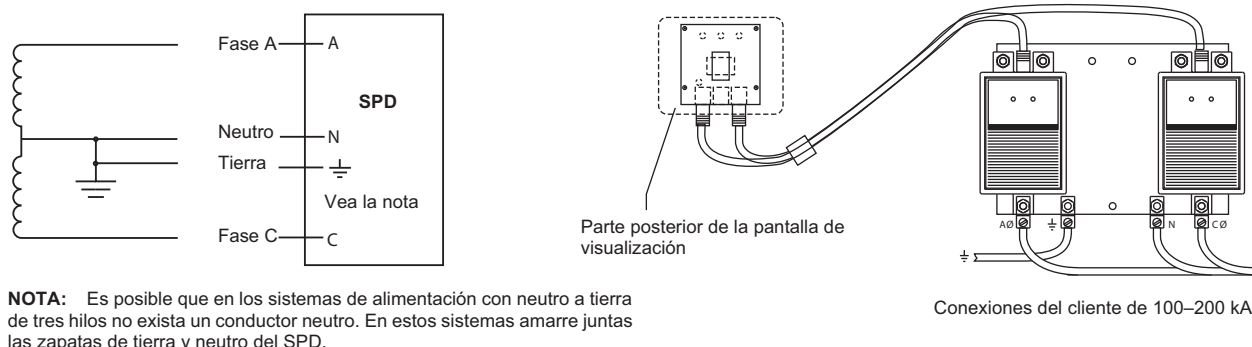
Figura 5: Instalación en estrella con conexión a tierra, de tres fases, 3 ó 4 hilos
