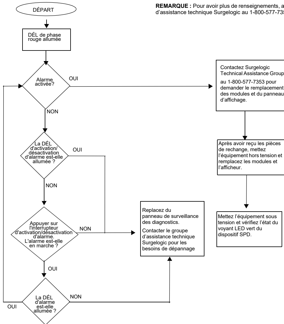
Figure 13 – Organigramme de dépannage
