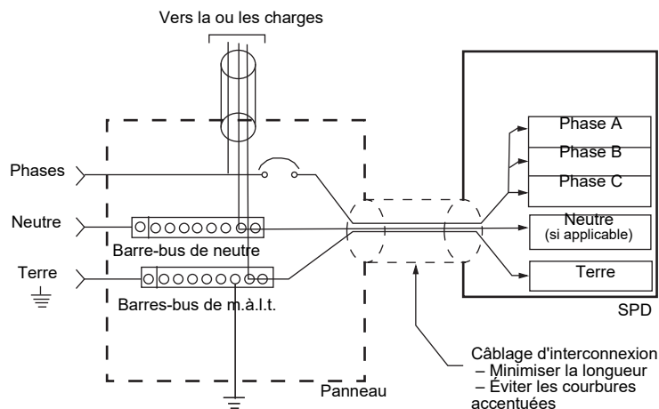
Figure 2 – Méthode de câblage du dispositif de protection contre les surtensions transitoires
