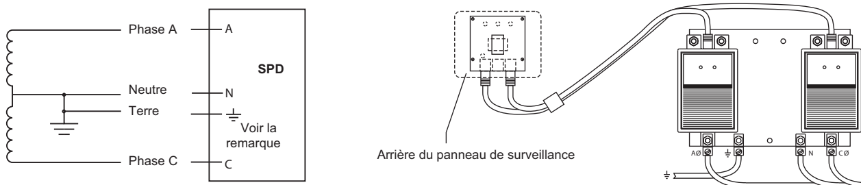
Figure 4 – Installation mise à la terre, monophasée à 3 fils
