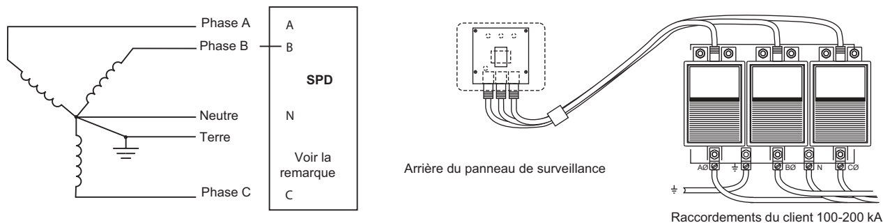
Figure 5 – Installation en étoile mise à la terre, triphasée à 3 ou 4 fils
