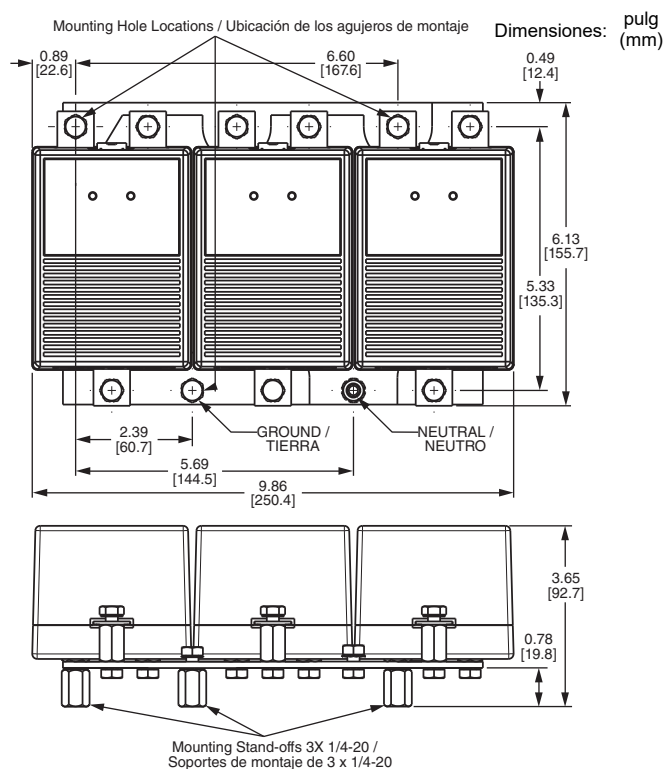
Figura 3: Dimensiones y montaje
