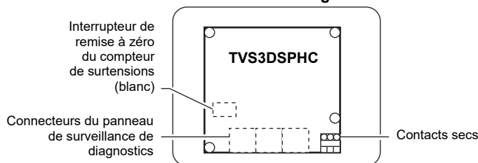
Figure 11 – Arrière de la carte de circuits des diagnostics
