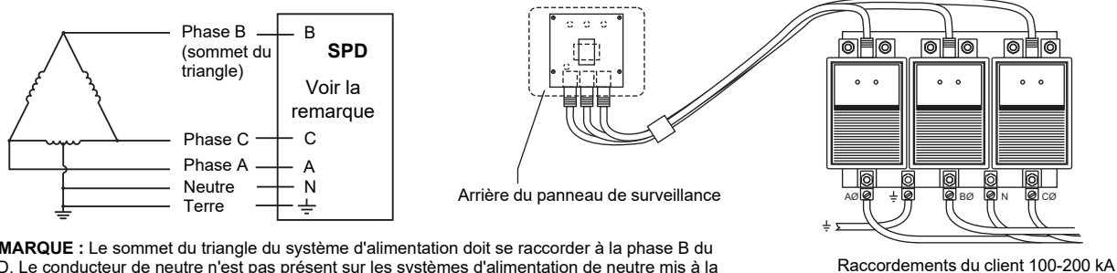
Figure 6 – Installation en sommet de triangle triphasée, à 3 ou 4 fils
