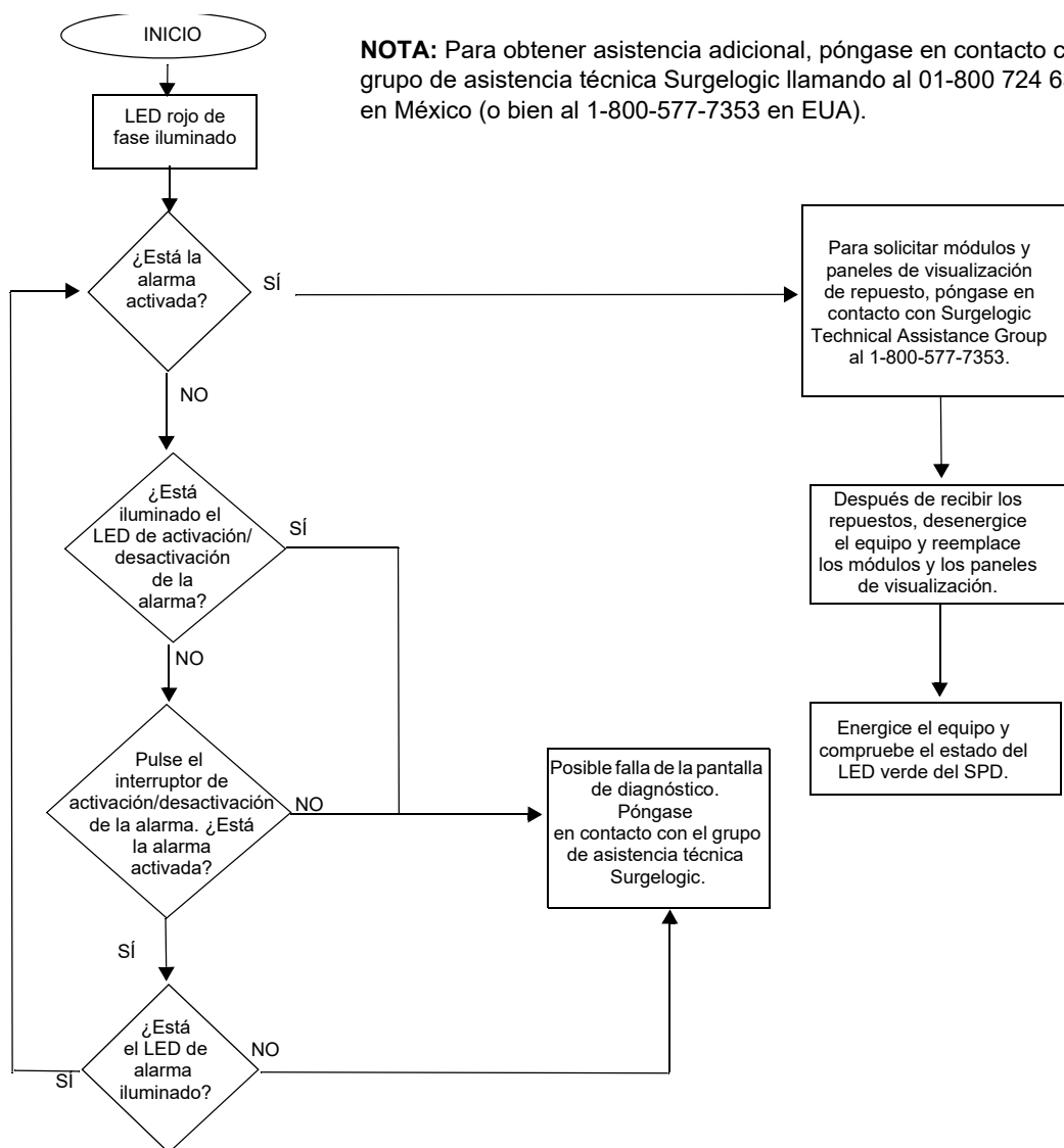
Figura 13: Cuadro de flujo de diagnóstico de problemas
