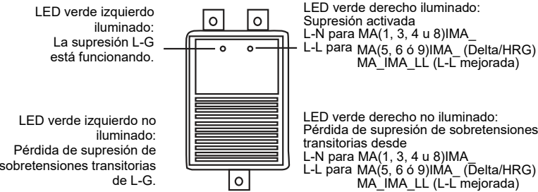
Figura 11: LED del módulo MA
