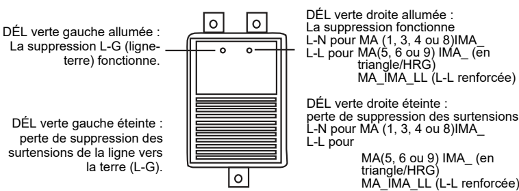
Figure 9 – DÉL du module MA
