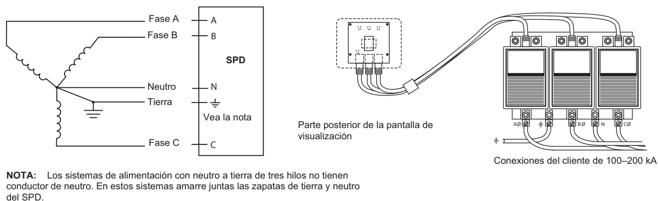
Figura 6: Instalación en delta con extremo alto de 3 fases, 3 ó 4 hilos
