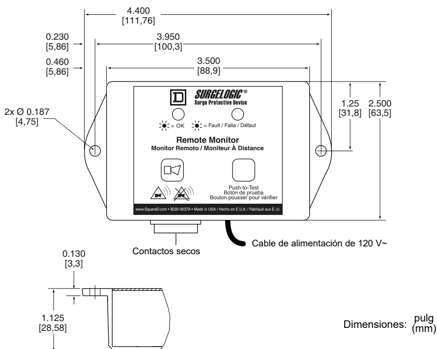
Figura 12: Monitor remoto opcional (TVS12RMU)
