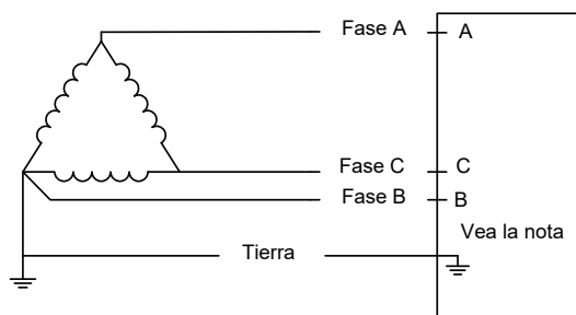
Delta con puesta a tierra de una fase (en esquina)
