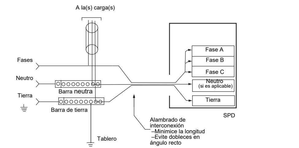
Figura 2: Prácticas de alambrado del dispositivo de protección contra sobretensiones transitorias
