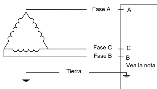
Delta sin puesta a tierra
