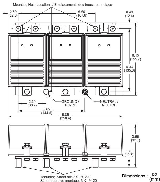
Figure 3 – Dimensions et montage
