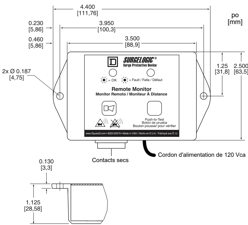
Figure 12 – Option de moniteur à distance (TVS12RMU)
