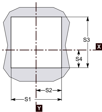
Front-Panel Cutout
