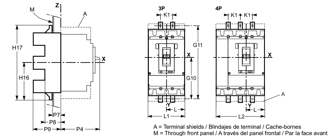
FIG. 6 : PowerPacT L-Frame Plug-In Circuit Breaker (On Base) / Interruptor automático enchufable PowerPacT marco L (sobre una base) / Disjoncteur enchufable PowerPacT à châssis L (sur socle)
