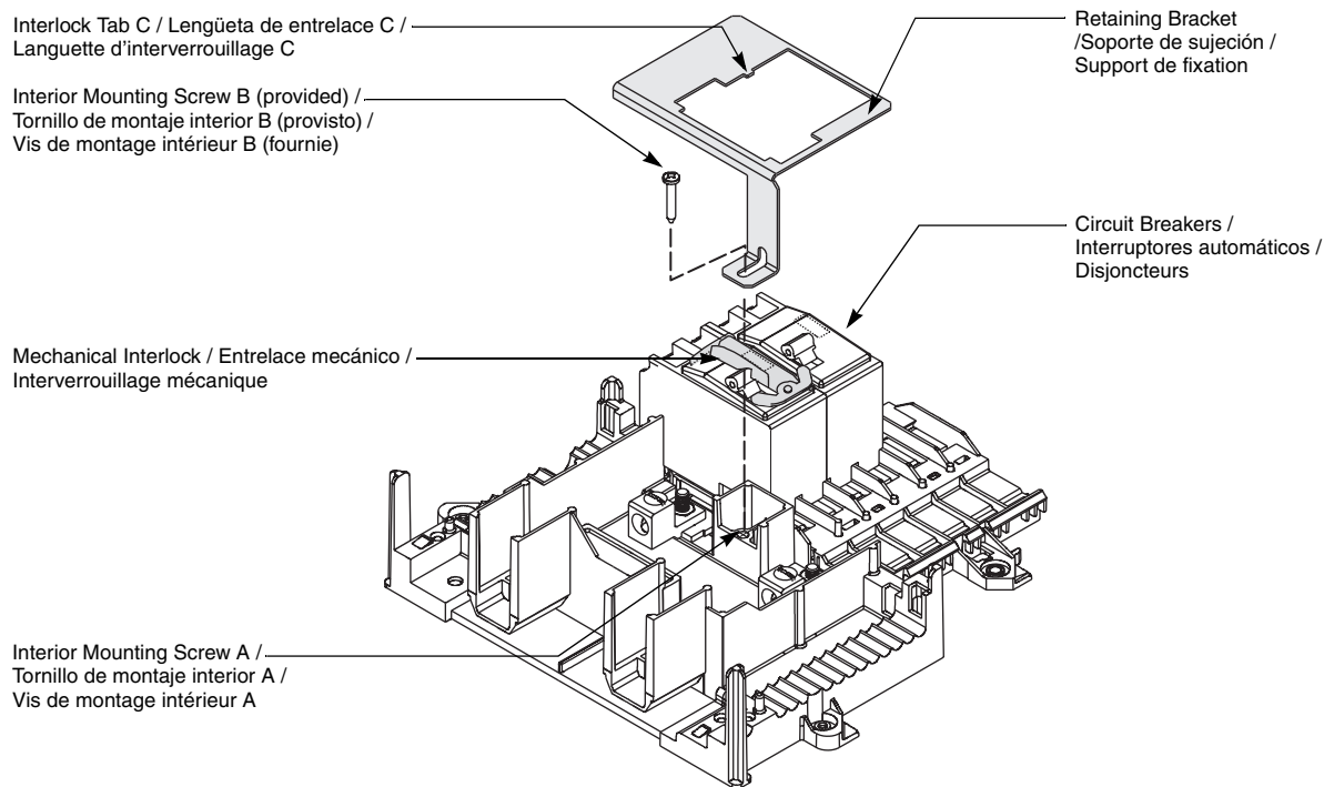
Figure / Figura / Figure 2 : Installing the Retaining Bracket / Instalación del soporte de sujeción / Installation du support de fixation
