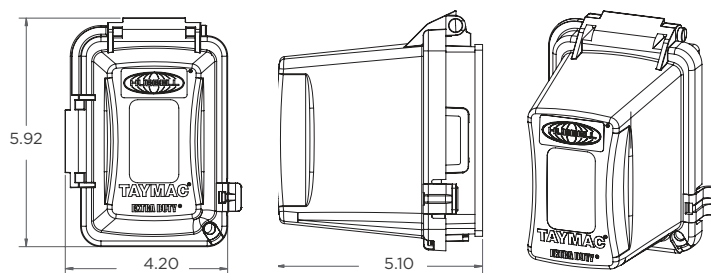
MM720
