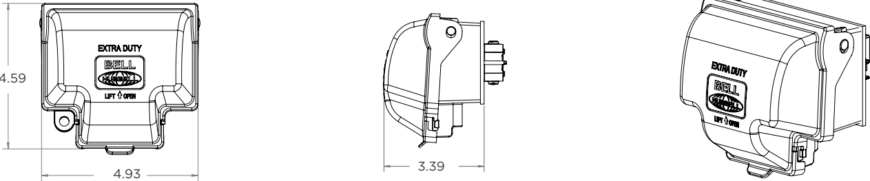
MD5802-O
