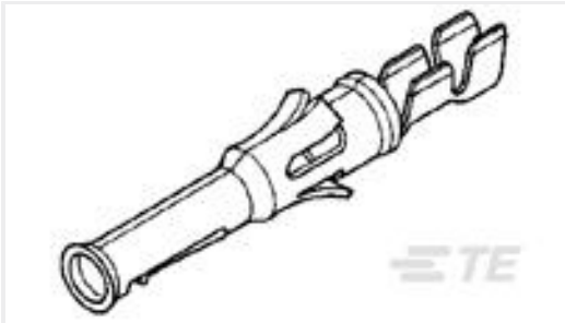
TE Part #66594-1 TYPE VI SKT CONT,MULTIMATE
