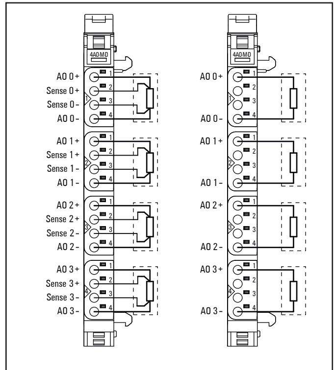
Connection diagram UR20-4AO-UI-16-M-DIAG
