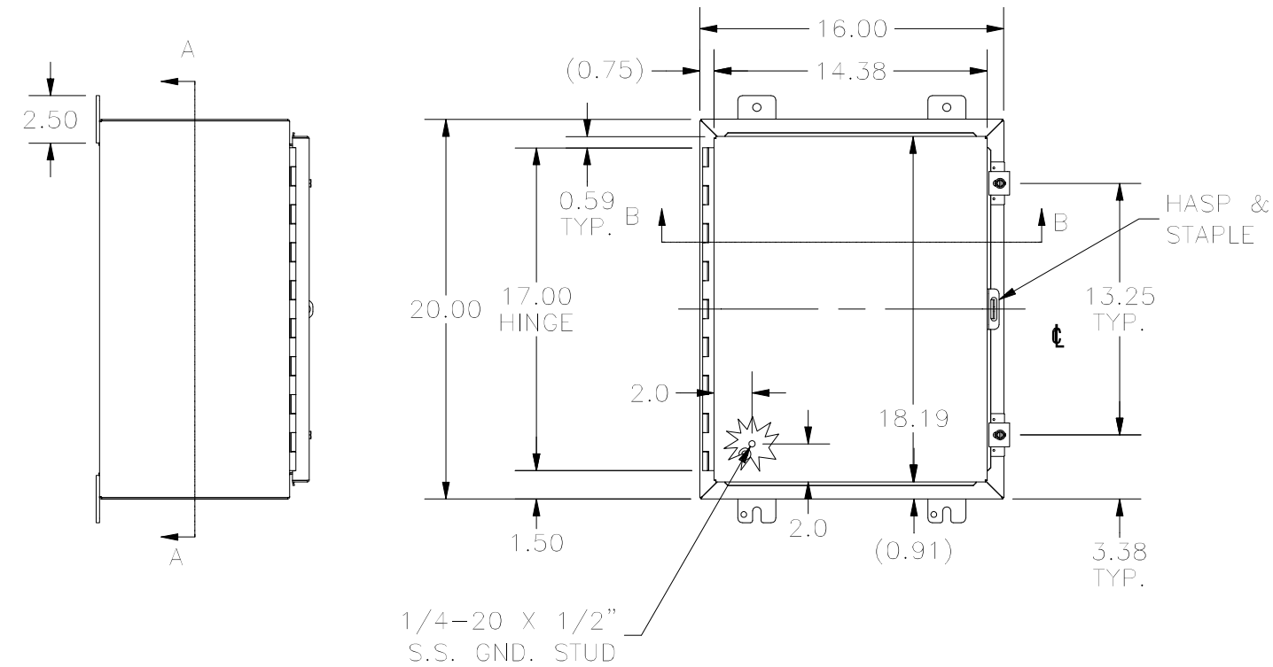
LEFT SIDE
